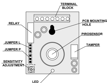
Рис 4 Вид печатной платы
