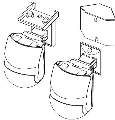
Рис 10 Варианты кронштейнов
