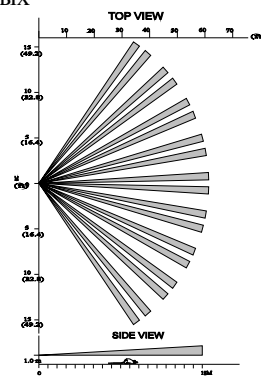
Рис 8 Диаграмма направленности линзы, обеспечивающей проход для животных
