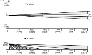
Рис 7 Диаграмма направленности «коридорной» линзы
