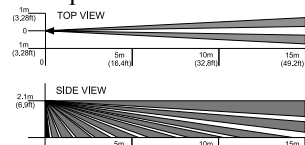
Рис 7 Диаграмма направленности «коридорной» линзы
